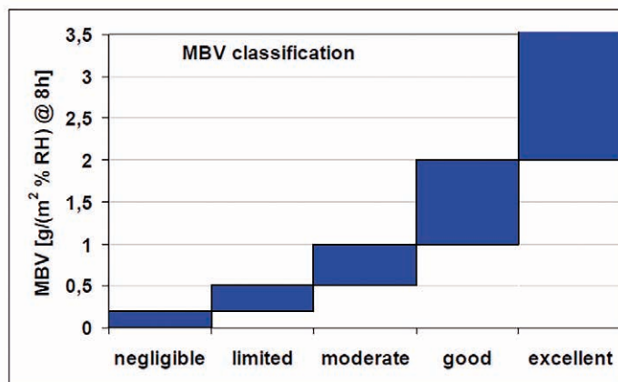
Figura 7.24. Clasificación de materiales según su potencial de amortiguamiento de humedad. Fuente: Nordtest Project.
