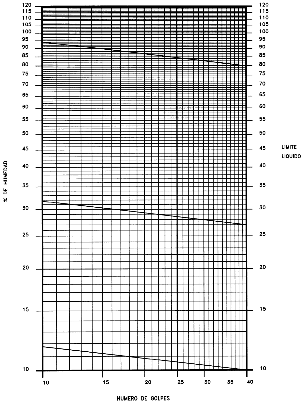
GRAFICA PARA LA DETERMINACION DEL LIMITE LIQUIDO
